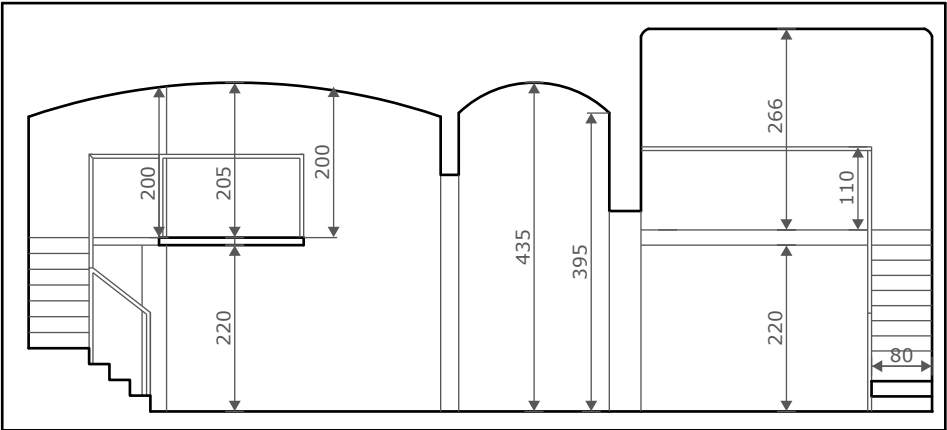
sezione A-A'
