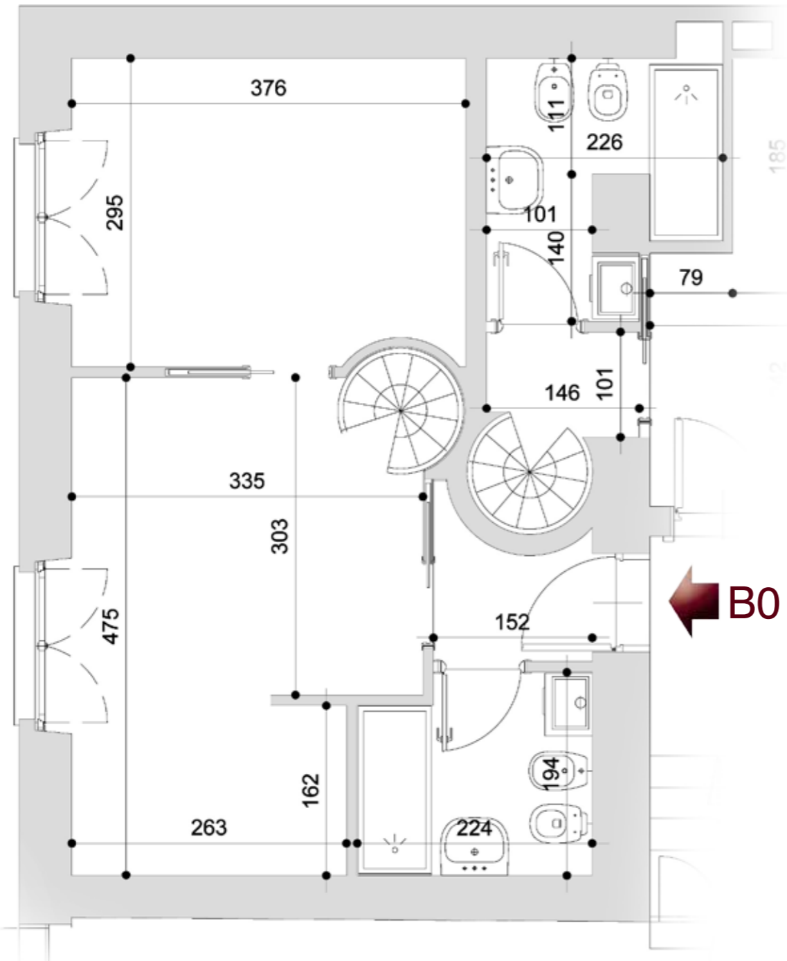
PIANO RIALZATO
