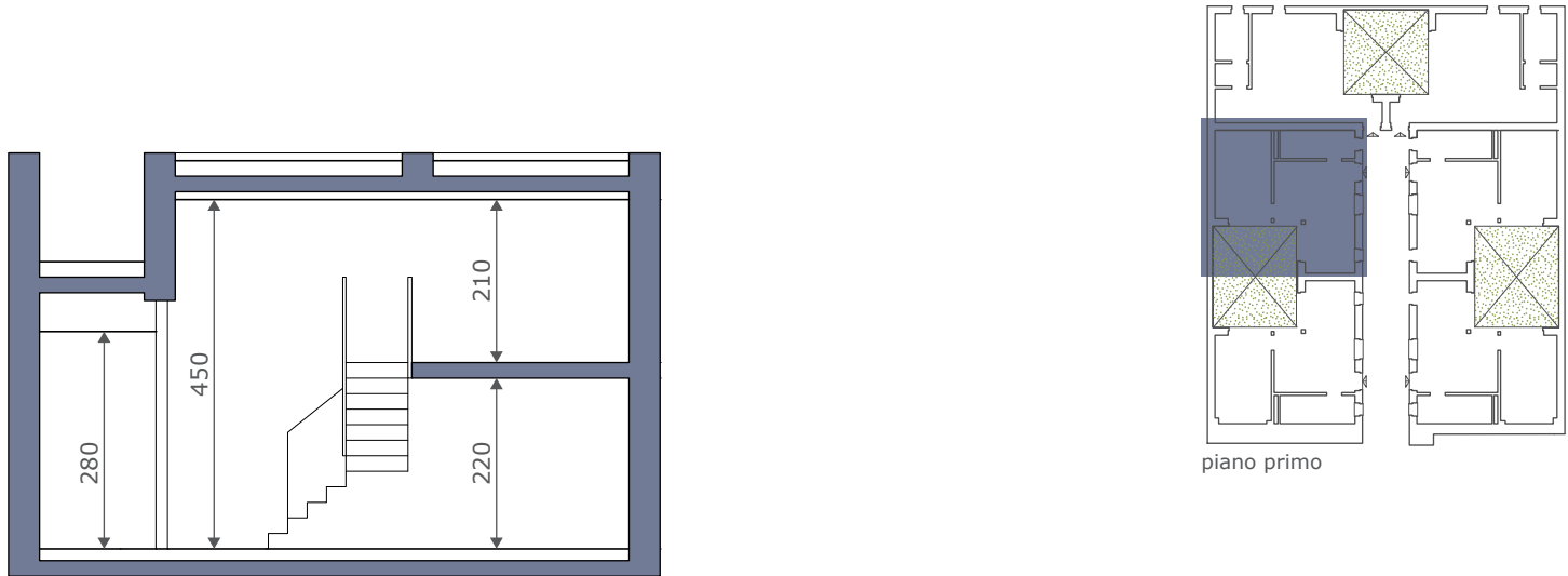
soppalco sezione
