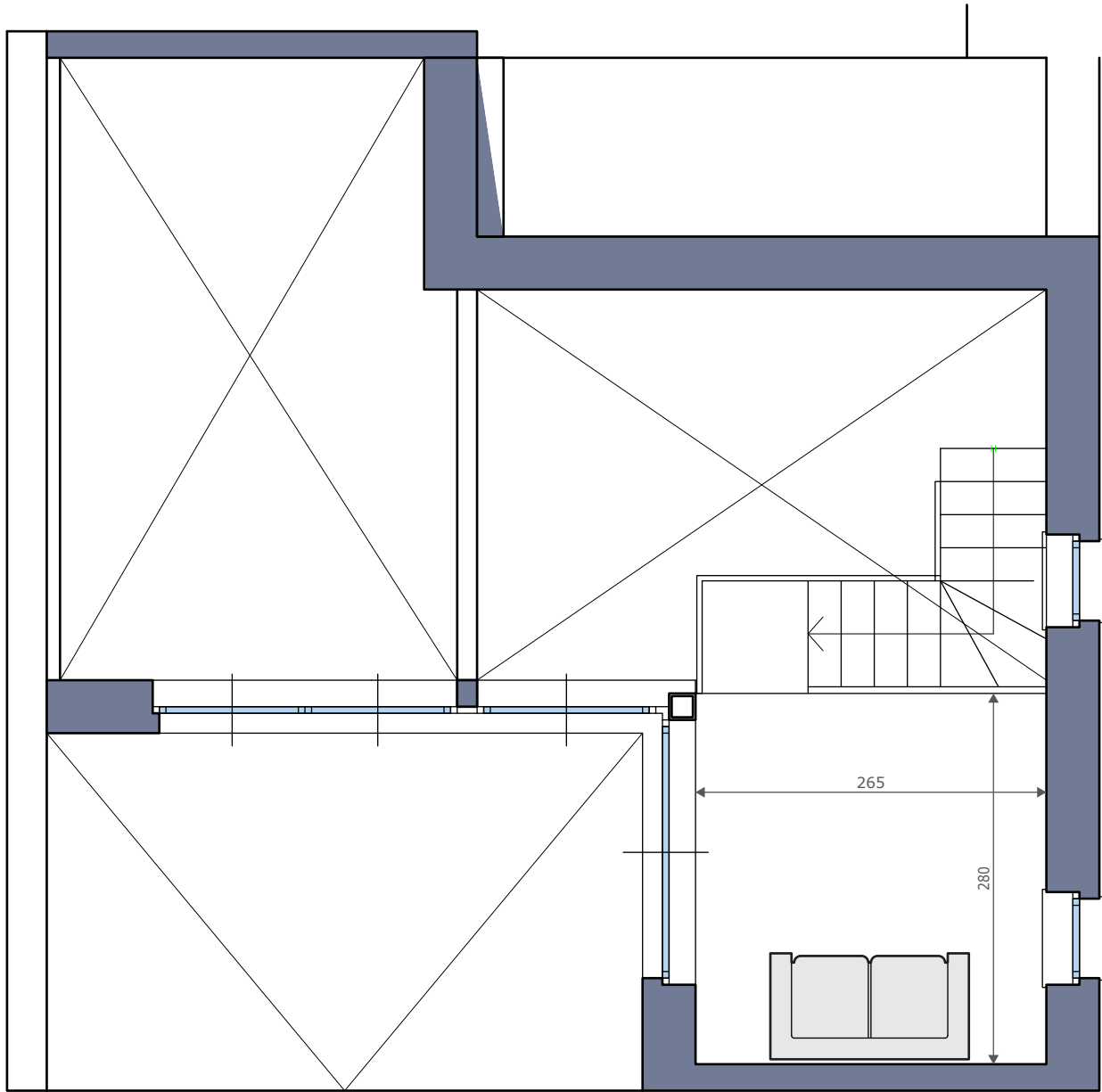
soppalco
