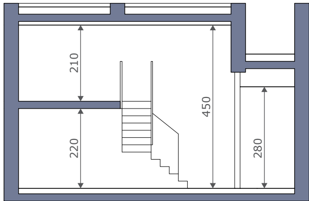
soppalco sezione
