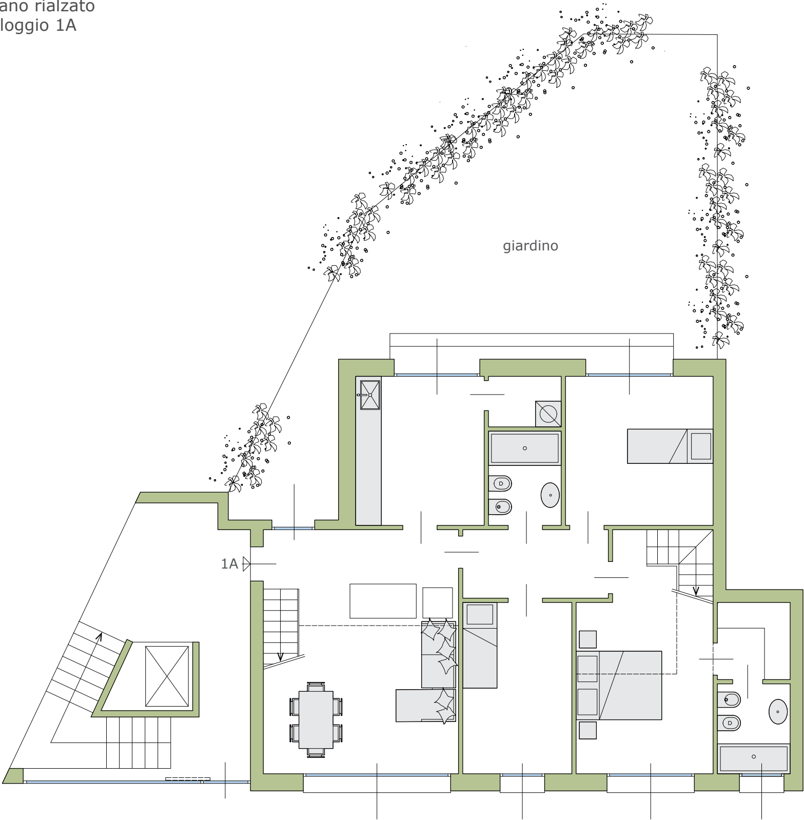
pianta piano rialzato
